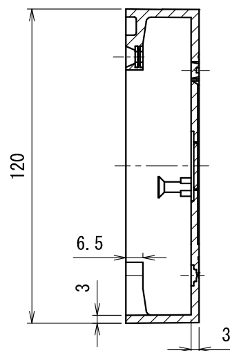
断面 A-A
